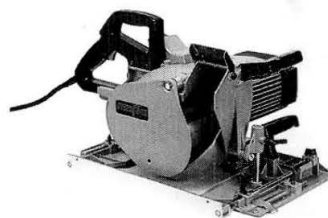
ZK 115 Fresatrice speciale per carpenteria in legno
