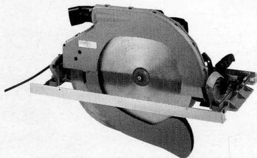
MKS 165 E Potente sega circolare; spessore mass. di taglio 165 mm orientabile da 0 - 60°, eccezionale per tagli lungovena.
