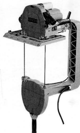
LS 103 Mortasatrice a catena per cave ed incastrati fino a prof., mass. 500mm
