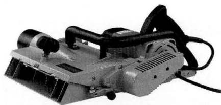
ZH 320 E Pialletto per travi in legno (largh. a piallare mm 320)
